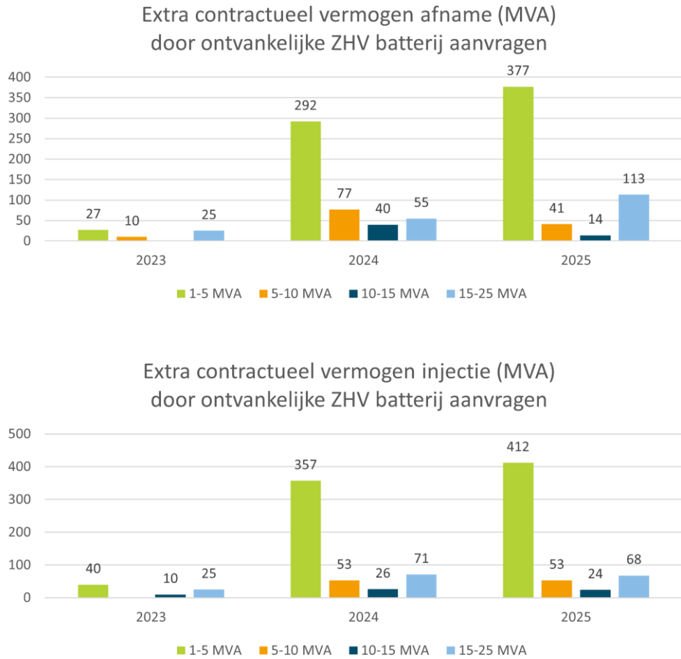
Figuur 37: aanvragen naar vermogen voor industriële batterijen.
