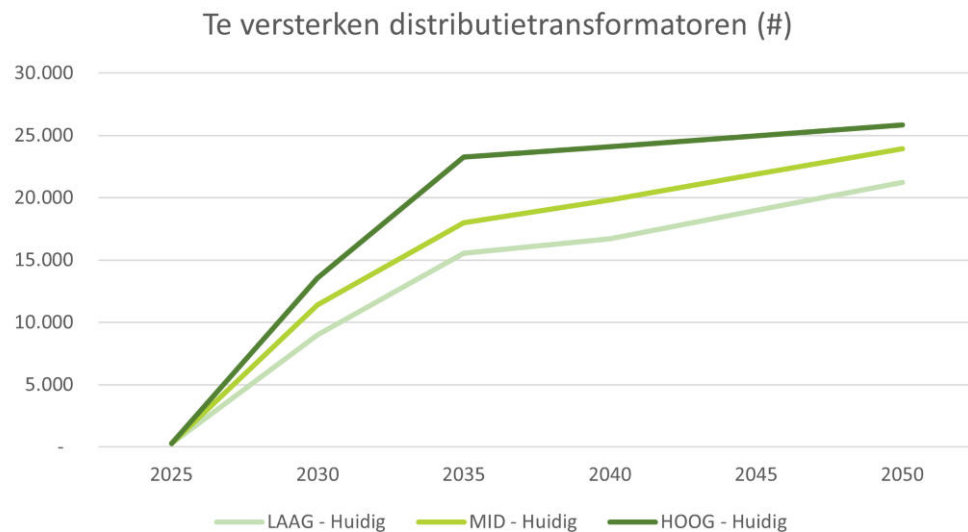
Figuur 48: het aantal transformatoren in congestie als niet zou worden geïnvesteerd.
