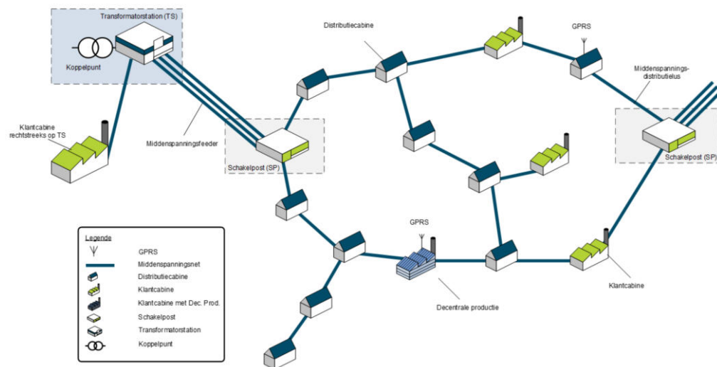
Figuur 2: schematische opbouw van een distributielus op middenspanning.
