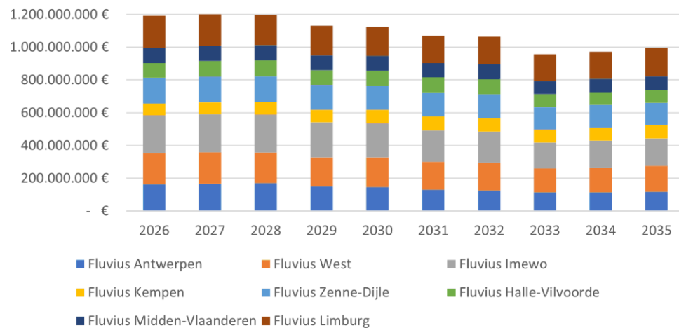
Bruto investeringen elektriciteit (excl. tussenkomst DNG)
