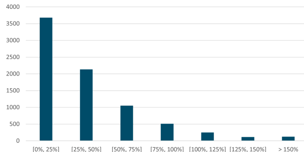
Figuur 52: piekbelasting distributielussen
